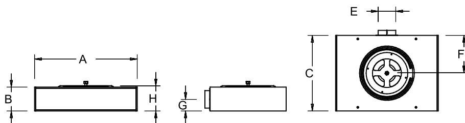
BBTQ33 nízký podstavec - rozměry (mm)
