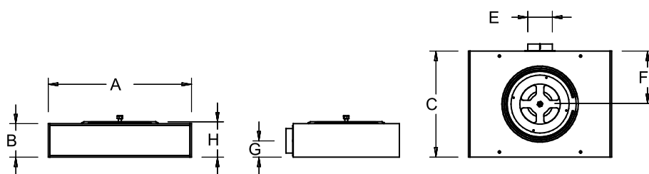
BBTQH43 nízký podstavec - rozměry (mm)
