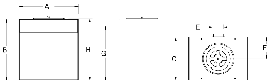
PLTQH13 podstavec se zásobníkem dřeva - rozměry (mm)
