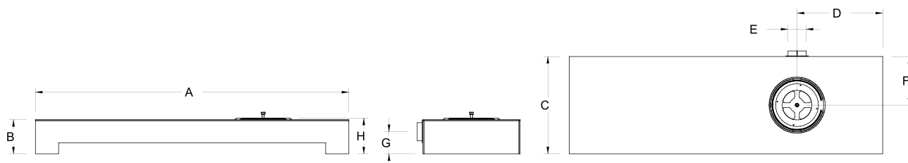
BLTQ/H Lavice L/P - rozměry (mm)
