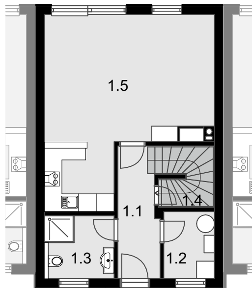
LEGENDA MÍSTNOSTÍ 1NP:
